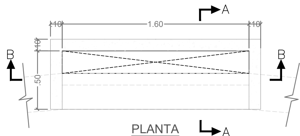
DETALLE TERMOSIFÓN ESC. 1_20
