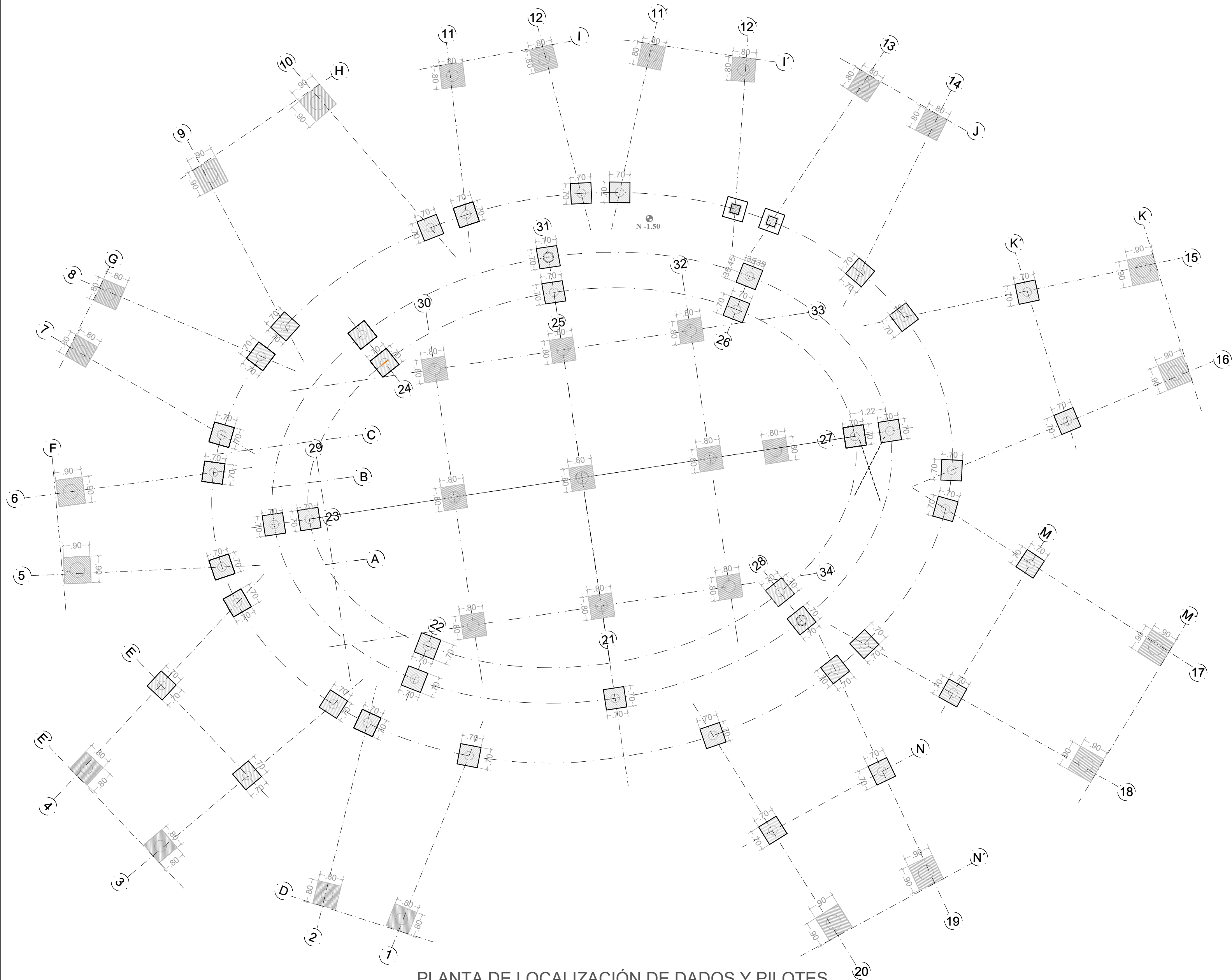
PLANTA DE LOCALIZACIÓN DE DADOS Y PILOTES ESC. 1:100
