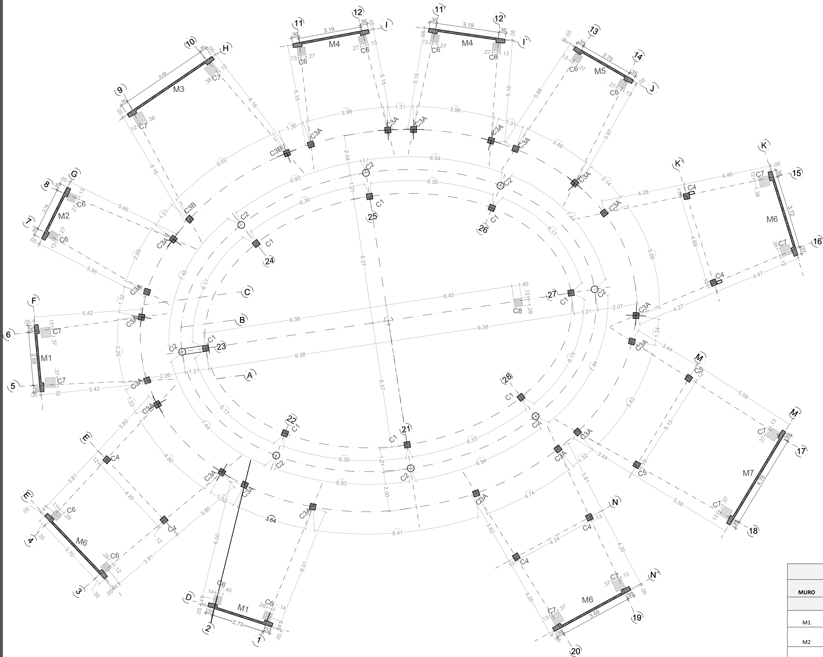
PLANTA DE LOCALIZACIÓN DE COLUMNAS Y MUROS ESC. 1:100
